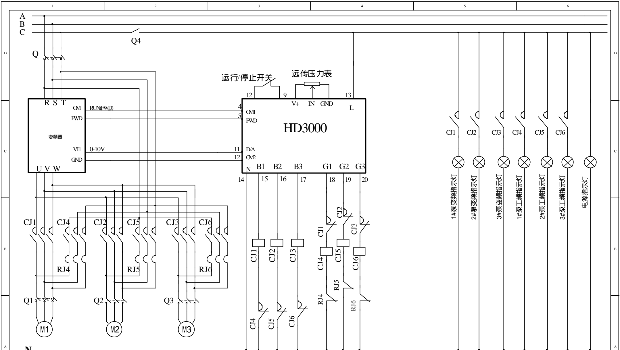
P03=7,三泵循环软起动控制
